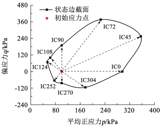
图10 垃圾土在 p - q 应力空间上的状态边界面 Fig. 10 State boundary surface of MSW in p - q stress space
