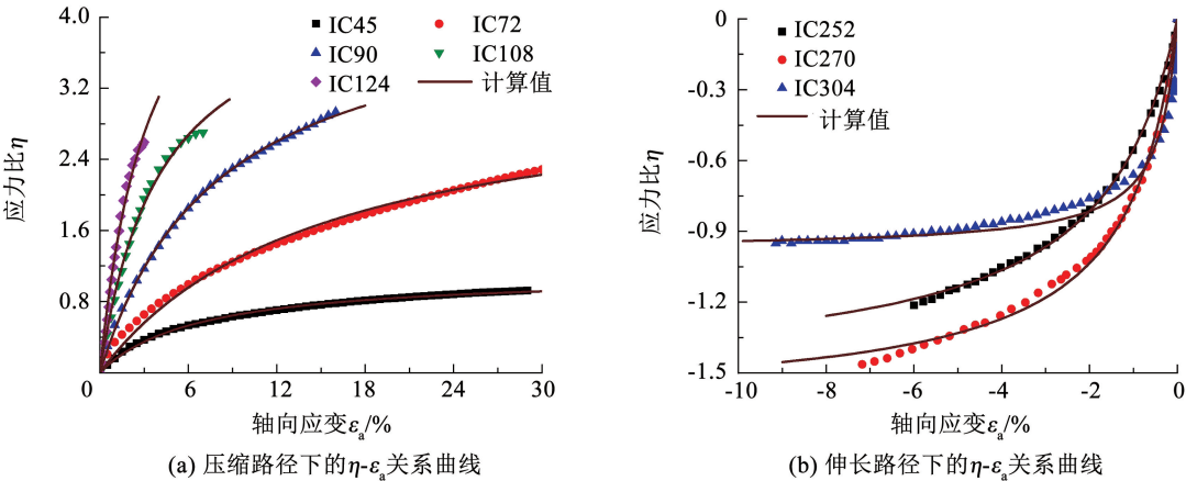
图 9 不同应力路径下垃圾土的应力比与轴向应变的关系
