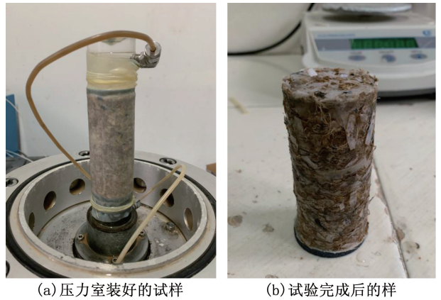
图 1 人工制备的垃圾土试样
