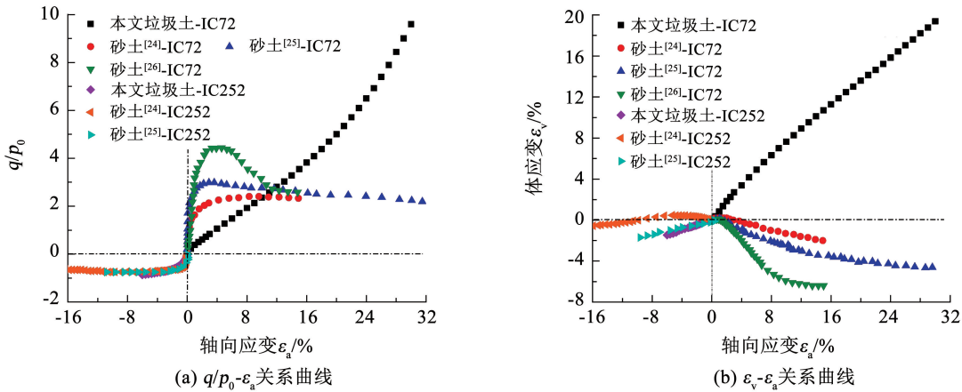
图 6 IC72 和 IC252 路径下垃圾土和砂土的应力 - 应变关系
