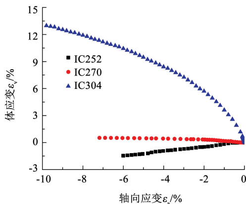
(b) \varepsilon_v - \varepsilon_a 关系曲线
