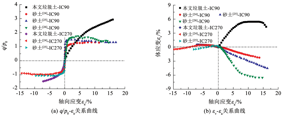
图 7 IC90 和 IC270 路径下垃圾土和砂土的应力 - 应变关系
