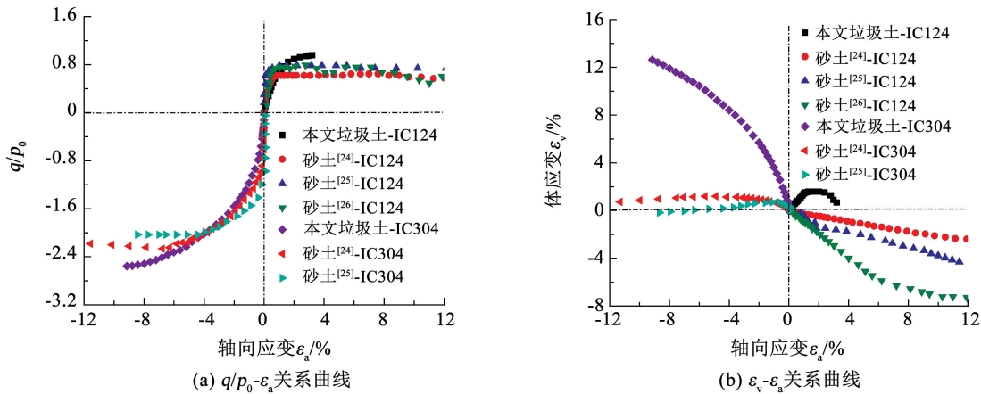
图 8 IC124 和 IC304 路径下垃圾土和砂土的应力 - 应变关系
