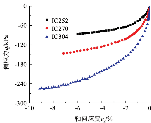
(a) q - \varepsilon_a 关系曲线
