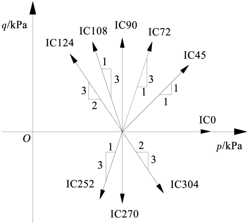
图 2 三轴应力路径试验方案
